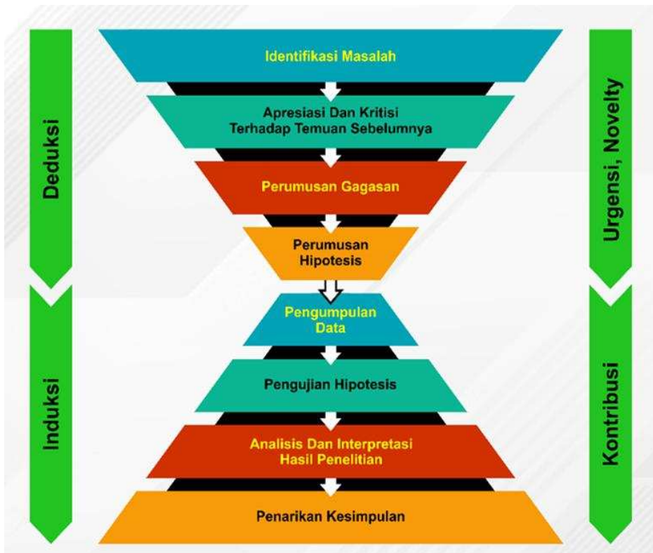
Gambar 1.1 Logika Deduktif-Induktif
